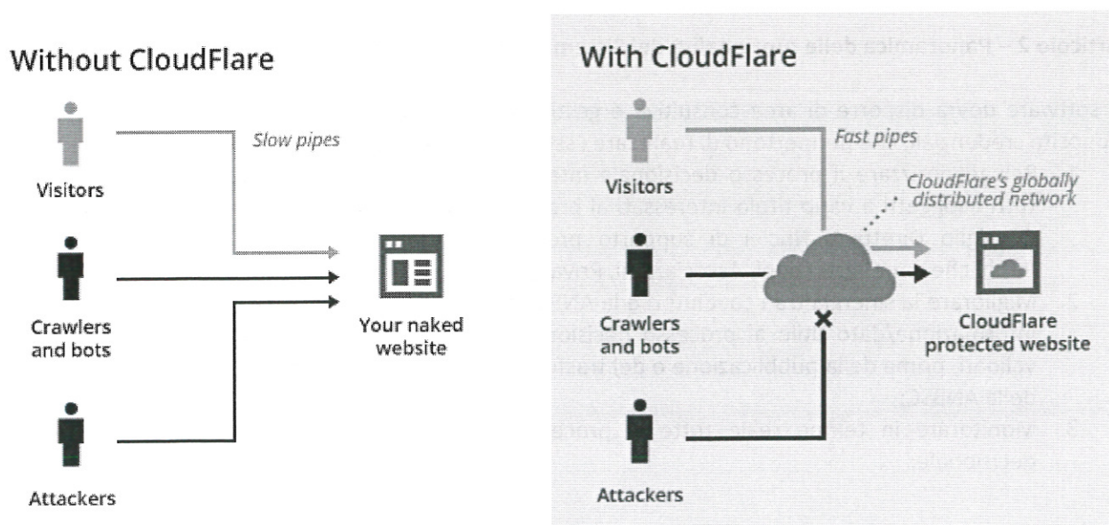
Funzionamento di CloudFlare
